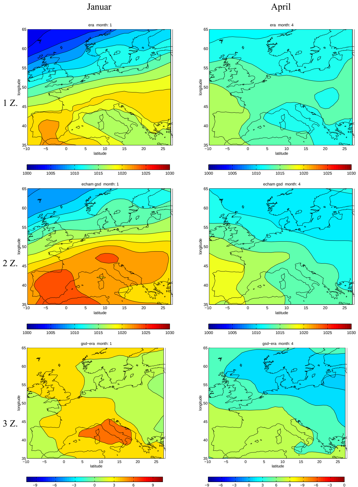
Abbildung 9: Vergleich von ERA40-SLP mit ECHAM-SLP. Mittelungsperiode: 1961–1990; erste Zeile : ERA40; zweite Zeile : ECHAM-GSD; dritte Zeile : Differenz ECHAM-GSD minus ERA40; links : Januar; rechts : April; [hPa].
