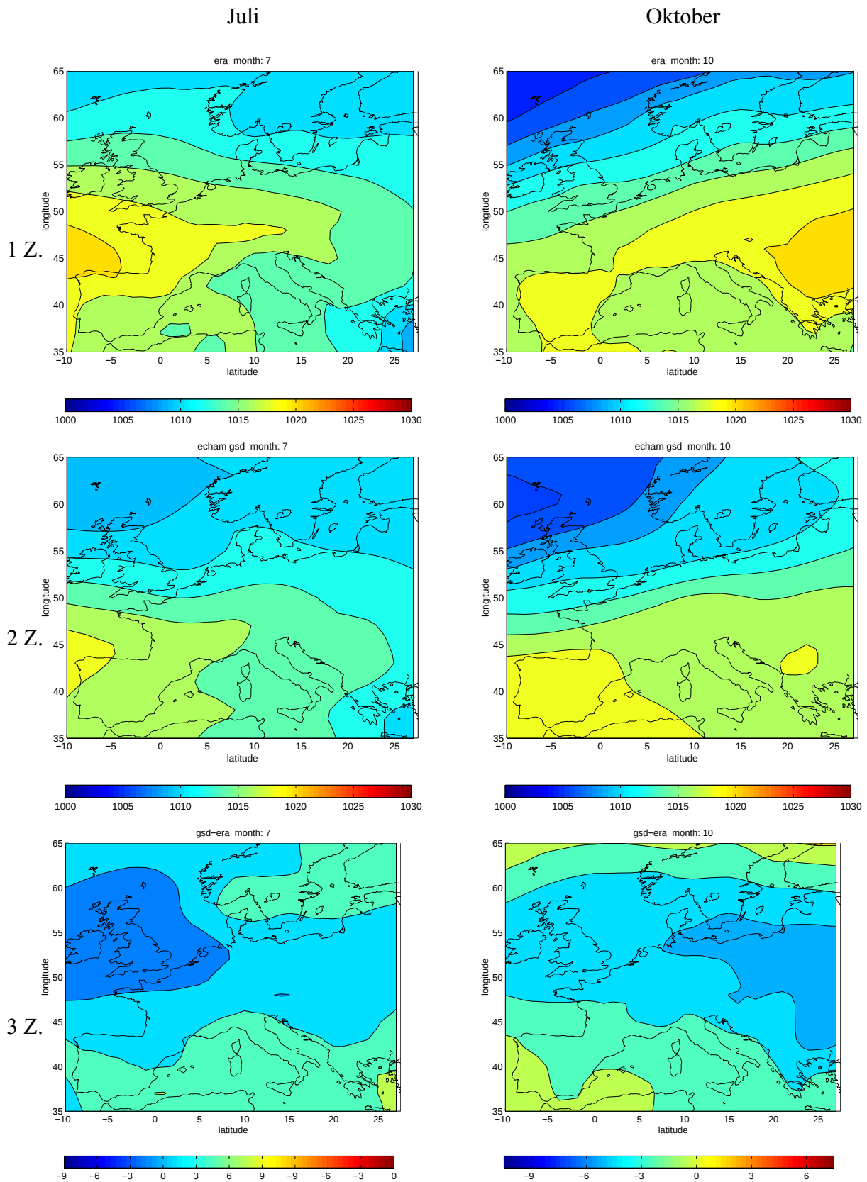
Abbildung 10: Vergleich von ERA40-SLP mit ECHAM-SLP. Mittelungsperiode: 1961–1990; erste Zeile : ERA40; zweite Zeile : ECHAM-GSD; dritte Zeile : Differenz ECHAM-GSD minus ERA40; links : Juli; rechts : Oktober; [hPa].
