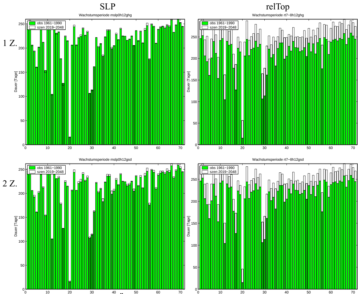
Abbildung 22: Modellierter Änderung der Wachstumsperiode an den Stationen. erste Zeile: GHG-Szenario, zweite Zeile: GSD-Szenario; grün: Beobachtung (1961–1990; Bergstationen sind dunkelgrün eingezeichnet); transparent: Szenario (2019–2048); linke Spalte: SLP, rechts: relative Topographie; x-Achse: Stationen von West nach Ost (siehe Abbildung 1), y-Achse: Länge der Wachstumsperiode [Tage]; (Vorsicht: Wertebereich ist je nach Prädiktor etwas unterschiedlich).
