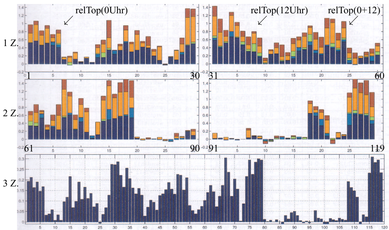
Abbildung 2: Graphische Darstellung des Validierungsexperiments. Zeile 1 und 2: x-Achse: Prädiktoren entsprechend ihrer Nummer in Tabelle 3, y-Achse: Leistung in den Saisonsen (dunkelblau: DJF, hellblau: MAM, grün: JJA, orange: SON, rot: Jahr); dritte Zeile: Leistung der Prädiktoren ohne Unterscheidung in Saisonsen, y-Achse: reskaliert.
