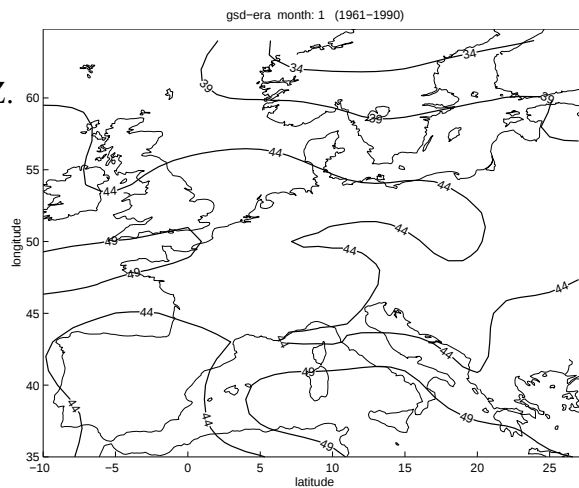
Abbildung 11: Vergleich von ERA40-relTop mit ECHAM-relTop. Mittelungsperiode: 1961–1990; erste Zeile: ERA40; zweite Zeile: ECHAM-GSD; dritte Zeile: Differenz ECHAM-GSD minus ERA40; links: Januar; rechts: April; [gpm].
