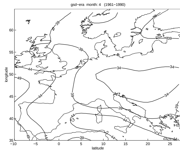
Abbildung 11: Vergleich von ERA40-relTop mit ECHAM-relTop. Mittelungsperiode: 1961–1990; erste Zeile: ERA40; zweite Zeile: ECHAM-GSD; dritte Zeile: Differenz ECHAM-GSD minus ERA40; links: Januar; rechts: April; [gpm].
