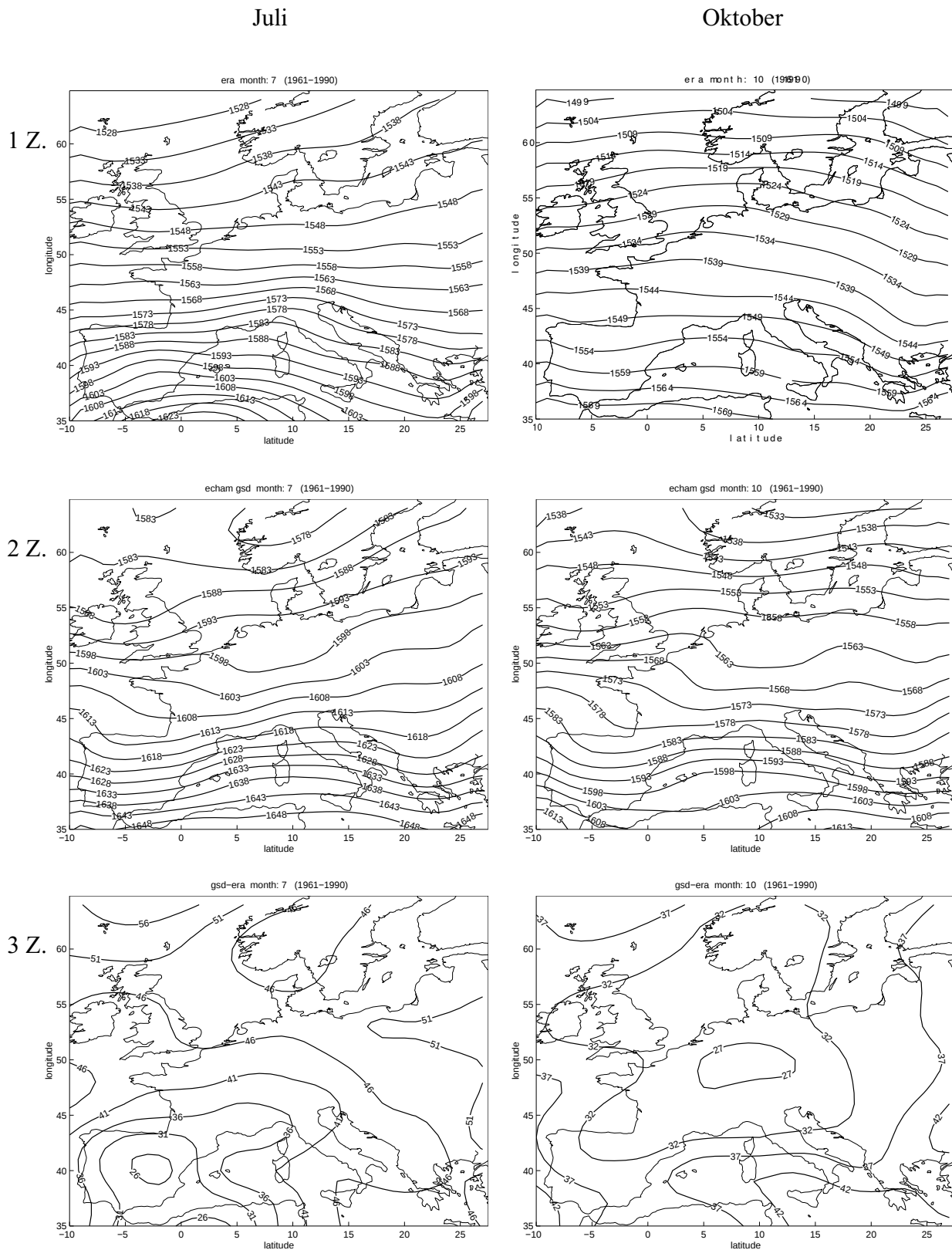
Abbildung 12: Vergleich von ERA40-relTop mit ECHAM-relTop. Mittelungsperiode: 1961–1990; erste Zeile: ERA40; zweite Zeile: ECHAM-GSD; dritte Zeile: Differenz ECHAM-GSD minus ERA40; links: Juli; rechts: Oktober; [gpm].
