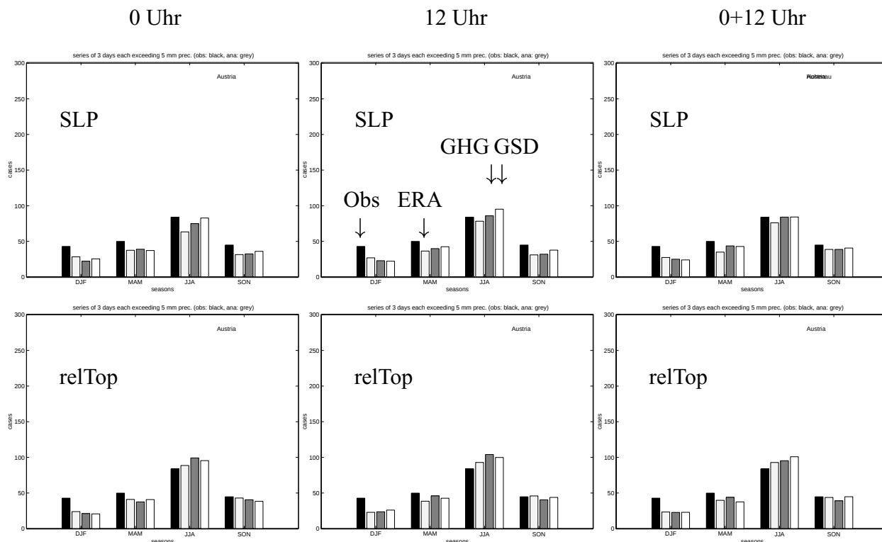
Abbildung 6: Episoden von drei Tagen mit Niederschlag (1958-2001) und ihre Reproduktion durch Analog-Methode + ERA und Analog-Methode + ECHAM; x-Achse: DJF, MAM, JJA, SON; y-Achse: Anzahl solcher Perioden an den Stationen; schwarz: Beobachtung; hellgrau: Analog-Methode + ERA40; dunkelgrau: Analog-Methode + ECHAM-GHG; weiss: Analog-Methode + ECHAM-GSD;
