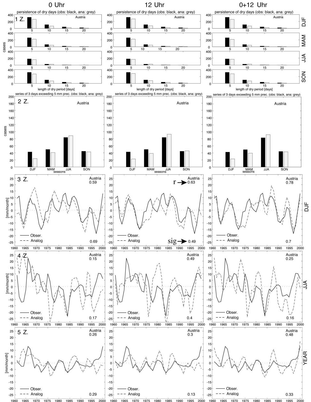
Abbildung 3: Reproduktion des Niederschlagsfeldes durch Analog-Methode+rel.Top. (1958–2001); schwarz : Beobachtung, weiss : Analog-Methode; erste Z. : saisonaler Zyklus von 5, 10, 15, 20 Tagen ohne Niederschlag; zweite Z. : saisonaler Zyklus von dreitägigen Niederschlagsereignissen; Z. 3 bis 5 : Simulation der Abfolge trockener und feuchter Saisonen (DJF/JJA/JAHR); rechts oben in den Bilder: r ; rechts unten : Prozentsatz an Stationen mit signifikantem r (Irrtumsw. 5 %).
