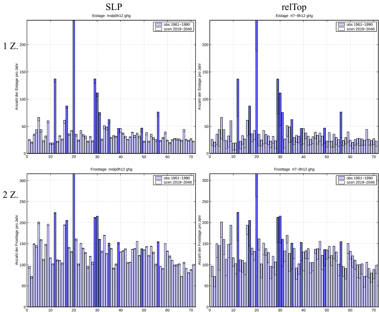
Abbildung 21: Modellierter Änderung von Eis- und Frostage in Österreich für das ECHAM-GHG-Szenario: erste Zeile: Eistage, zweite Zeile: Frostage; blau: Beobachtung (1961–1990; Bergstationen sind dunkelblau eingezeichnet), transparent: Szenario (2019–2048); linke Spalte: SLP ist Prädiktor, rechts: relative Topographie ist Prädiktor. x-Achse: Stationen von West nach Ost (siehe Abbildung 1), y-Achse: Zahl der Frost-/Eistage. (Vorsicht: Wertebereich ist bei den Eis- und Frostage unterschiedlich).
