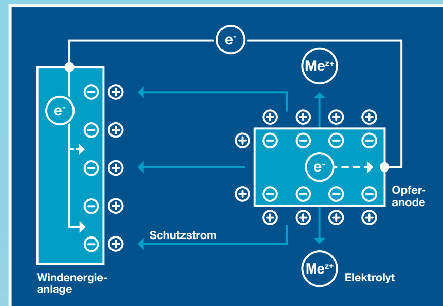
Schematischer Aufbau
